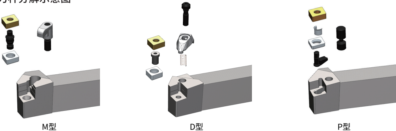
刀杆分解示意图
